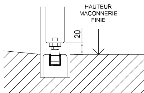
F GUIDAGE SUR BALCON AVEC PASSAGE HANDICAPE
