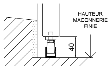
G GUIDAGE SUR BALCON SANS SEUIL DEBORDANT
